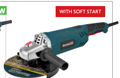
Angle grinder • 2200W • Ø230mm • 6500rpm
